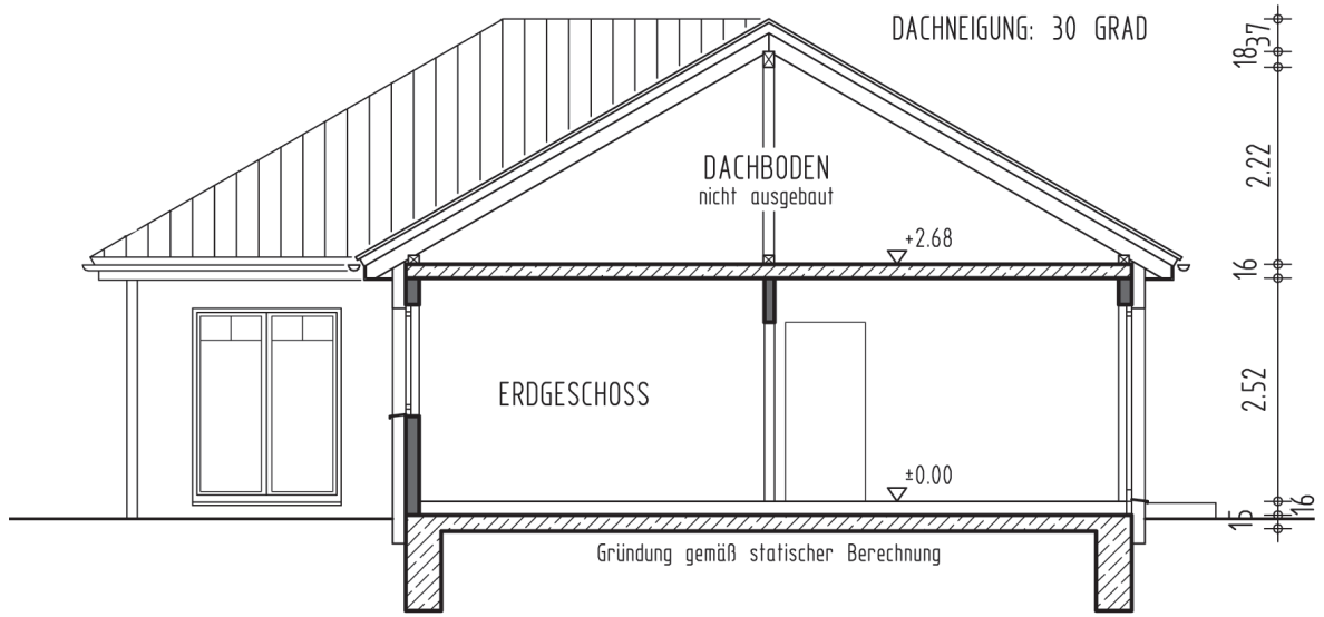
Schnitt
